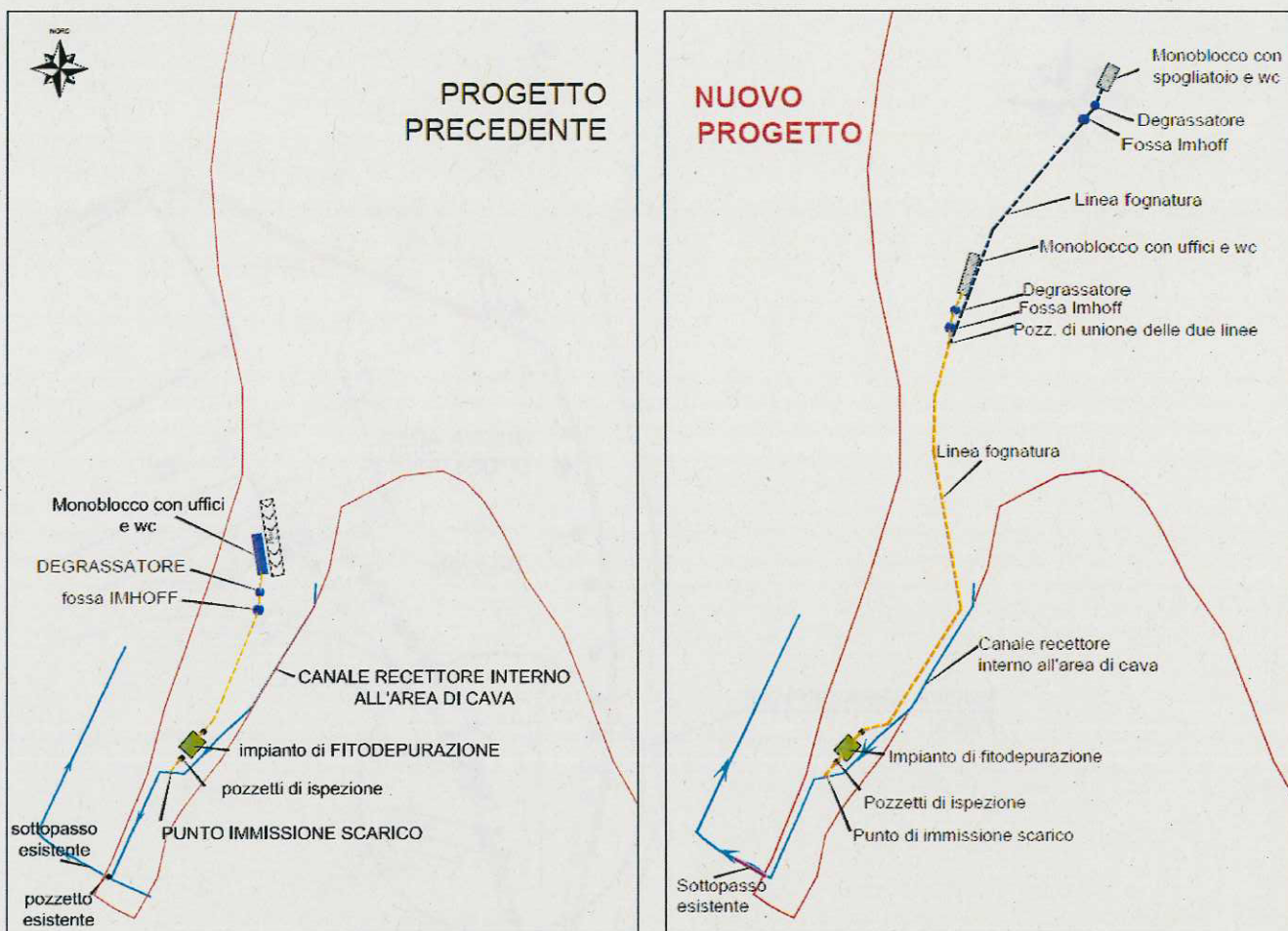
Figura B.2 Schematizzazione per confronto progetti
