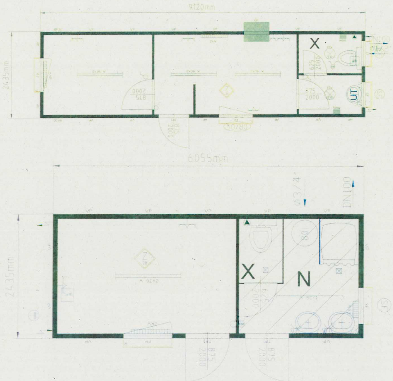
Figura B.3 Planimetrie dei nuovi container per uffici e spogliatoi
