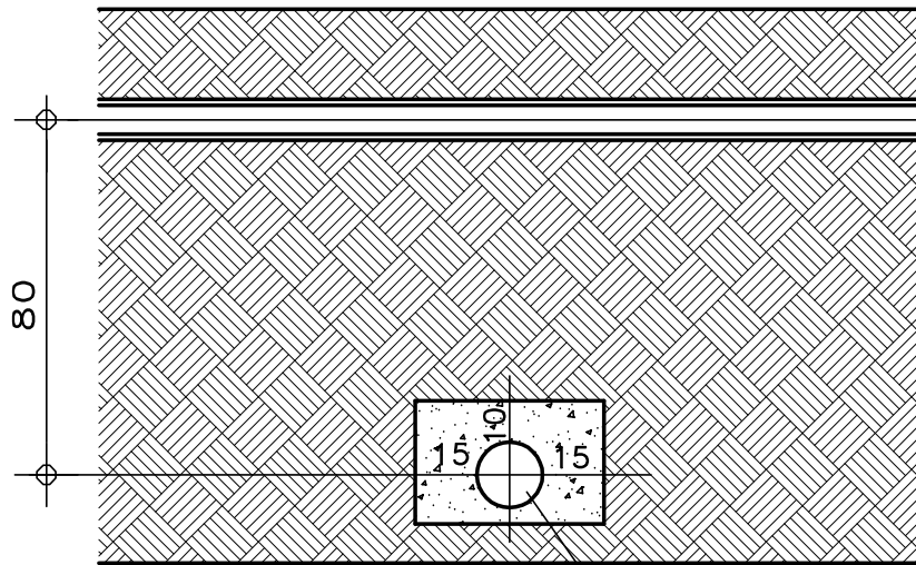
TUBO FOGNATURA rinfiancato in calcestruzzo
