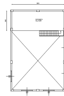
PIANO PRIMO _scala 1:100_
