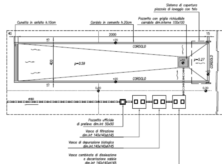
PARTICOLARE DEL SISTEMA DI TRATTAMENTO PER DELLE ACQUE PROVENIENTI DALLA PIAZZOLA LAVAGGIO CAMION Scala 1:50
