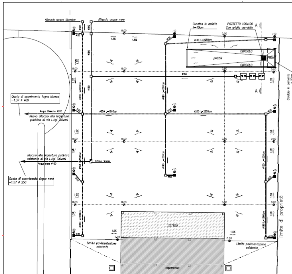
PLANIMETRIA FOGNATURA Scala 1:100
