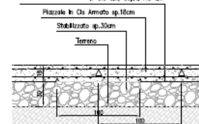
SEZIONE TIPO PIAZZALE
