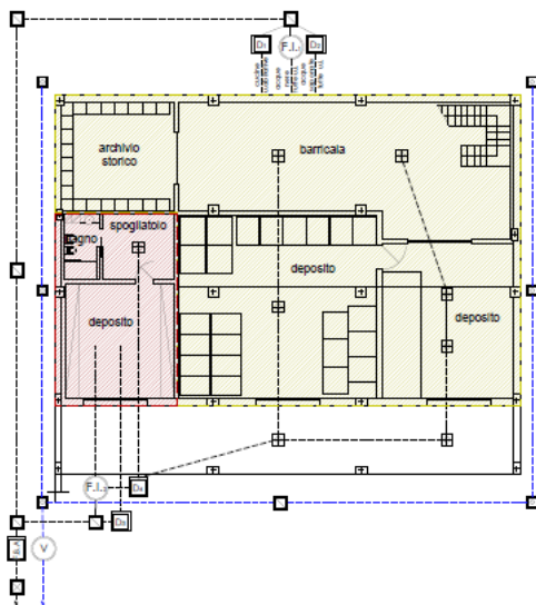
Pianta piano interrato - scala 1:200
