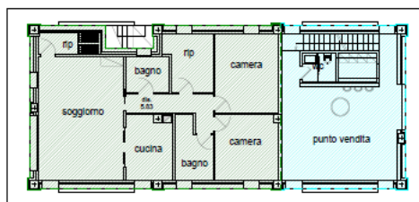
Pianta piano terra - scala 1:200
