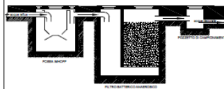
Sezione schema depurazione acque reflue scala 1:25
