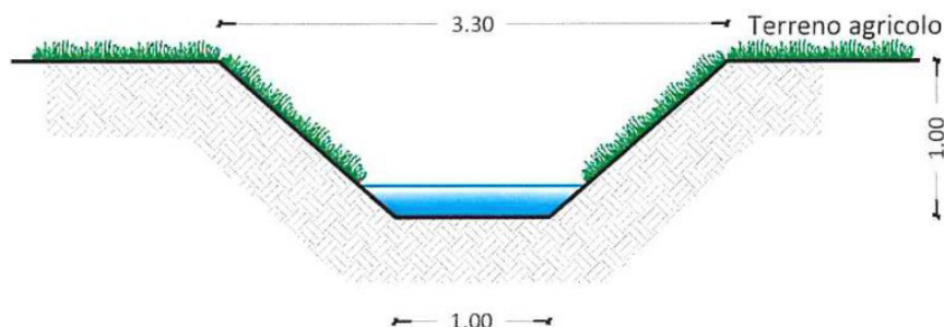
Stato Attuale - Scala 1:50
