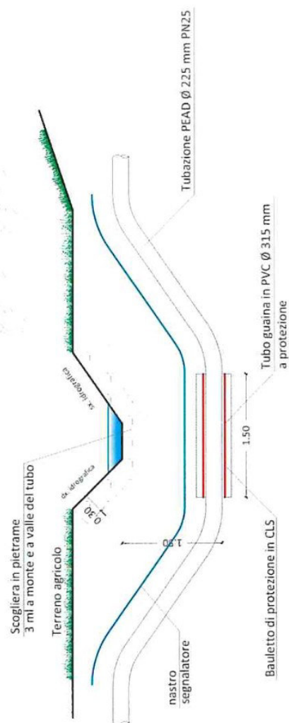
Stato di progetto - Scala 1:50
