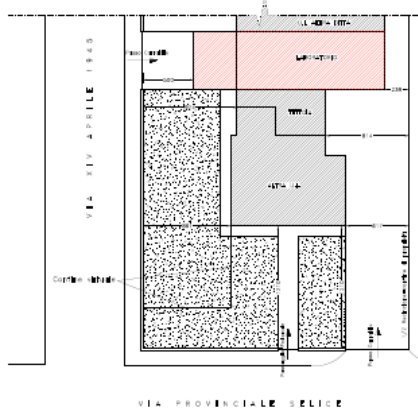
SVILUPPO PLANIMETRICO Scala 1:200
