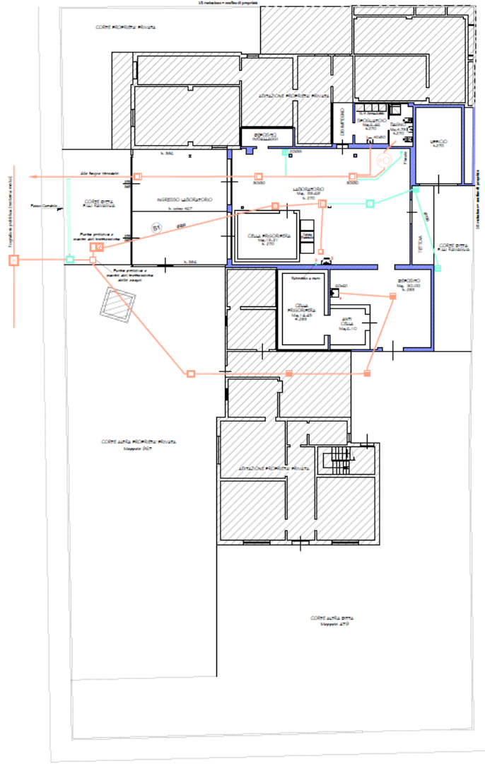
PIANO TERRA - Scala 1:100
