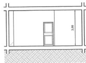
SEZIONE A-A SCALA 1:100
