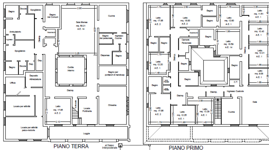
PIANO PRIMO
