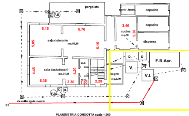
PLANIMETRIA CONDOTTA scala 1:200
