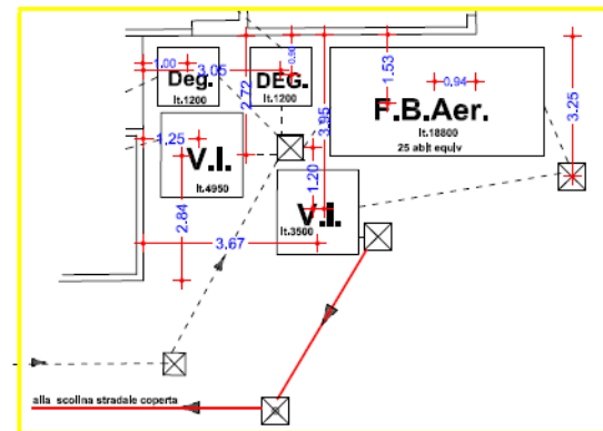
PARTICOLARE scala 1:100
