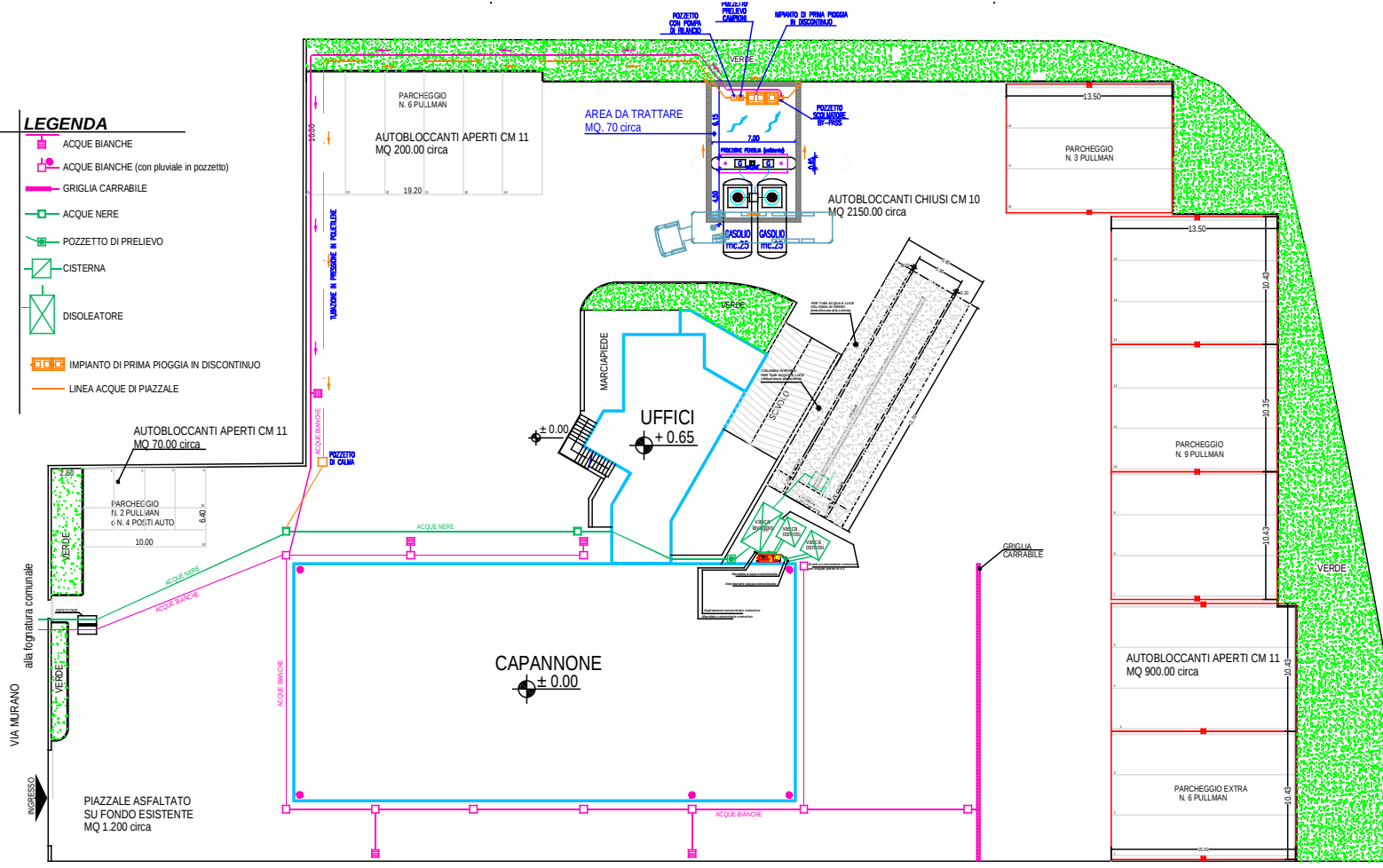
PLANIMETRIA 1:200
