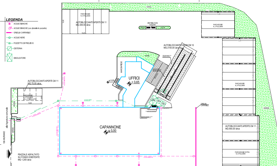
PLANIMETRIA 1:200
