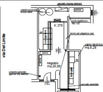
pianta piano terra - stato comparato controsoffitto in cartongesso h. 2,75 lay-out arredi ed attrezzature
