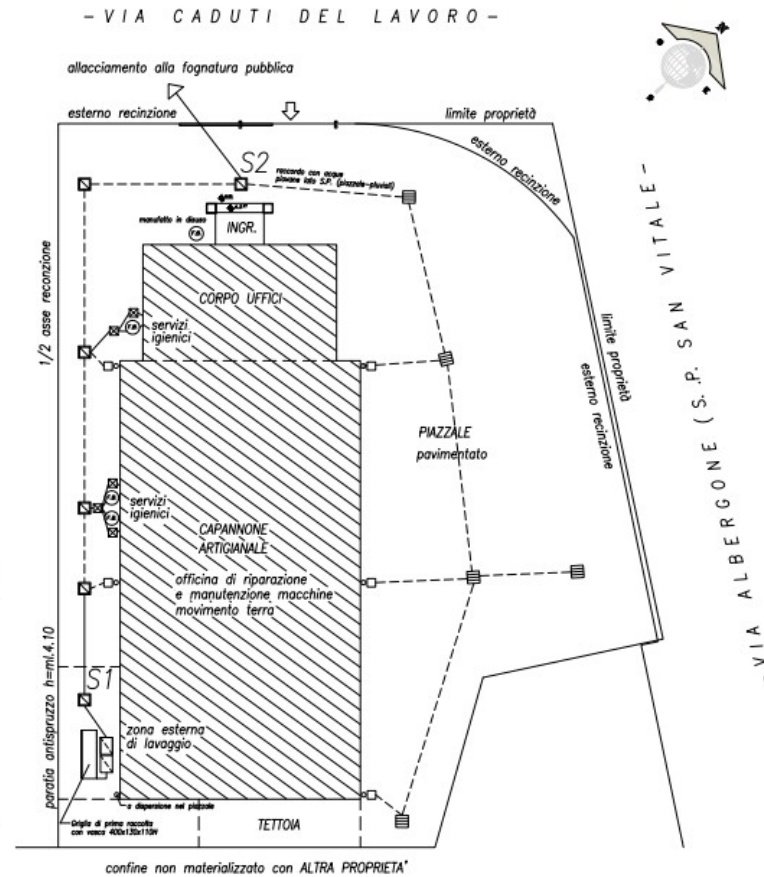
PLANIMETRIA RETE FOGNARIA scala 1 : 200
