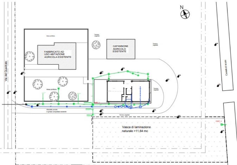
FOGNATURE DI PROGETTO Scale 1:25
