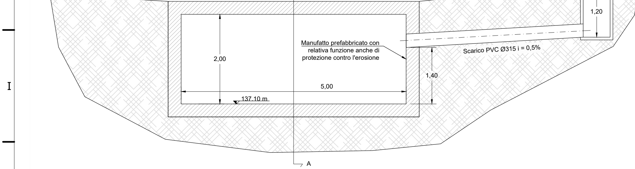
Profilo longitudinale Rio Mercato Scala H:500 V:250
