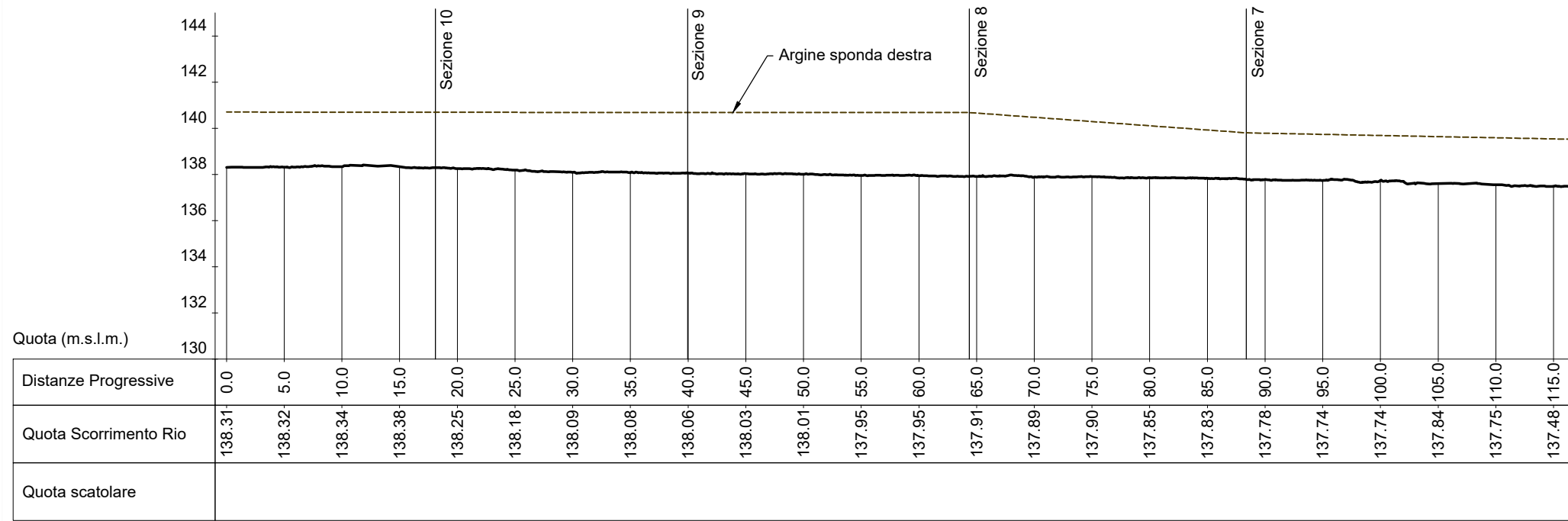
Profilo longitudinale Rio Mercato Scala H:500 V:250
