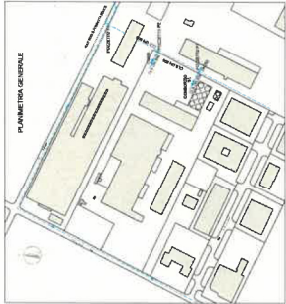
SCHEMA TRACCIATO COLLETTORE PRIVATO ORA CUT (EX CNH, EX BENATI)
