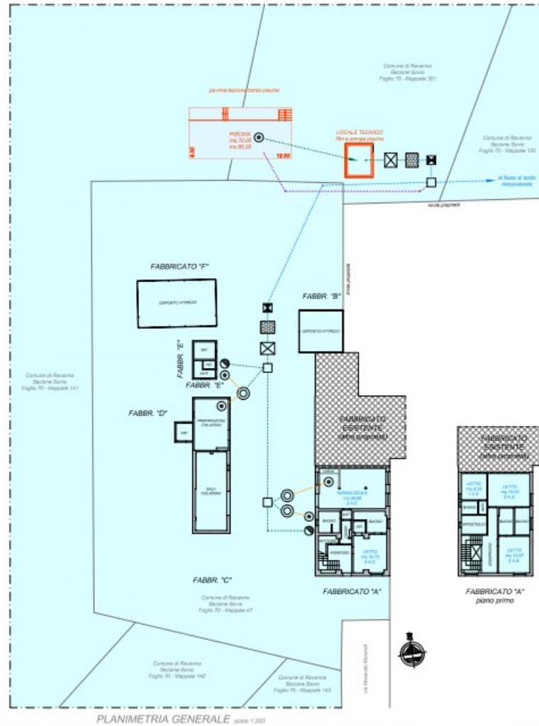
PLANIMETRIA GENERALE scala 1:300
