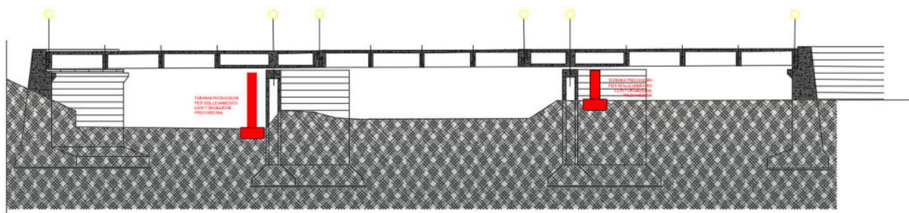
Figura 3 - Configurazione per il sollevamento d'impalcato con Torrini di presa
