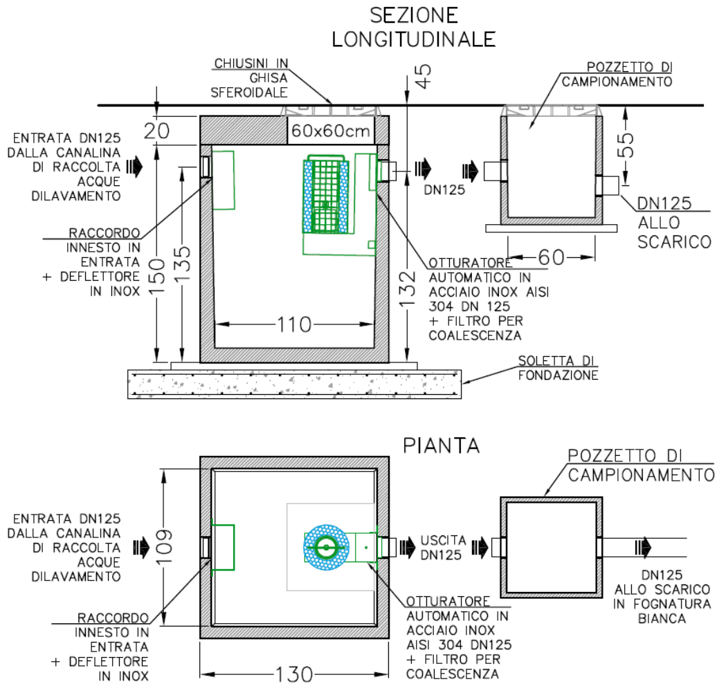
POZZETTO DISOLIATORE Scala 1:50
