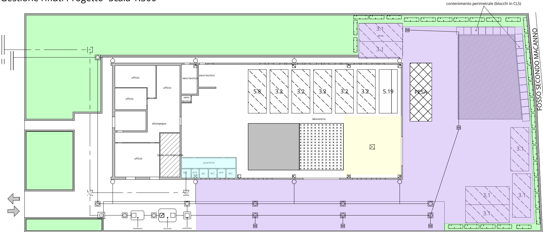
Gestione rifiuti Progetto- Scala 1:300
