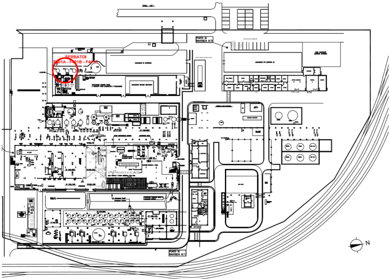
Cambio destinazione d'uso serbatoi – localizzazione all'interno dell'impianto FXXI
