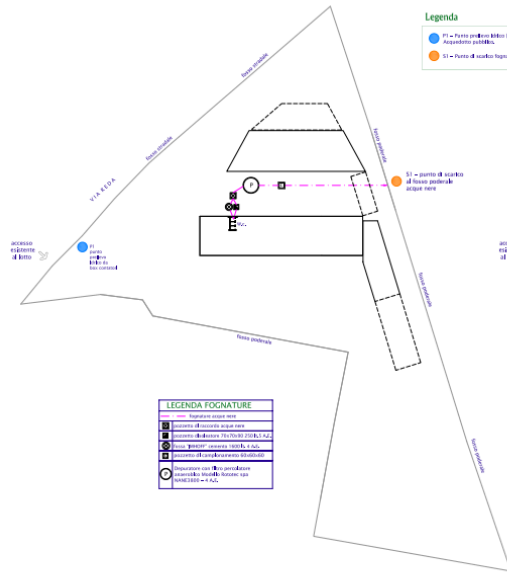
Schema rete fognaria - ACQUE NERE (come da autorizzazione allo scarico n°131/2019)
