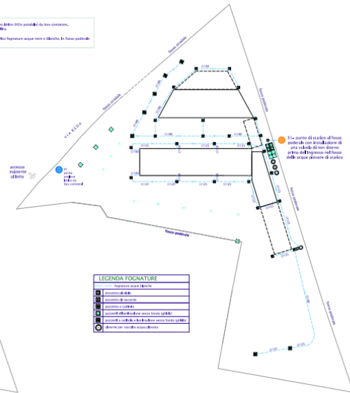
Schema rete fognaria - ACQUE CHIARE
