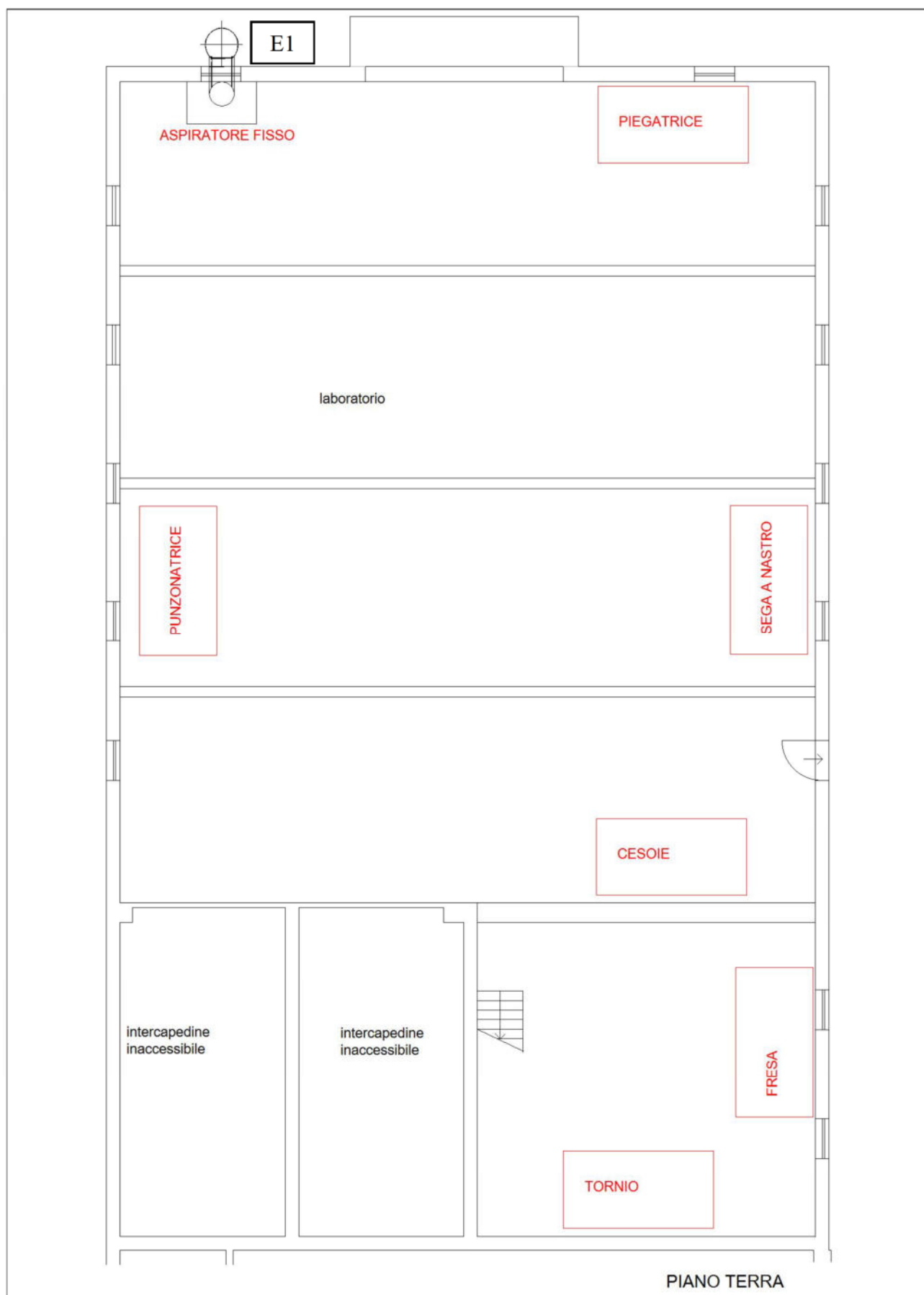
Figura 3: Planimetria del laboratorio con posizione dei macchinari
