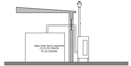
SEZIONE
