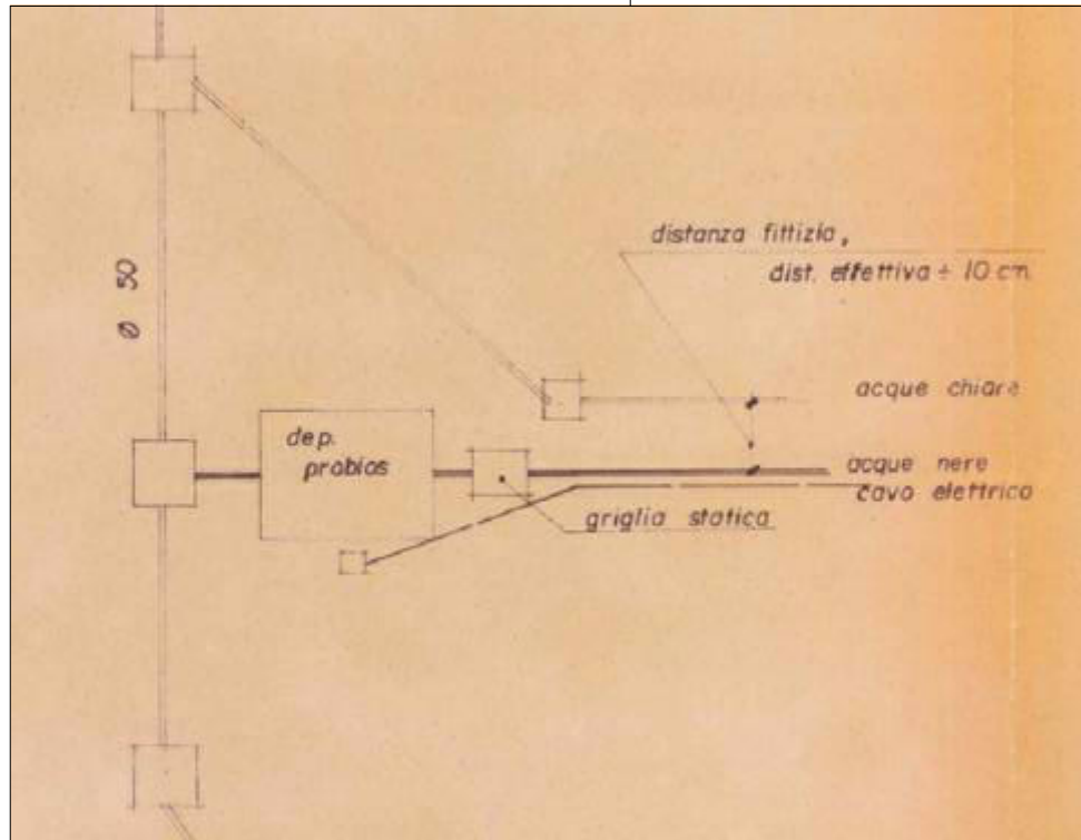
SCHEMA IMPIANTO ATTUALE
