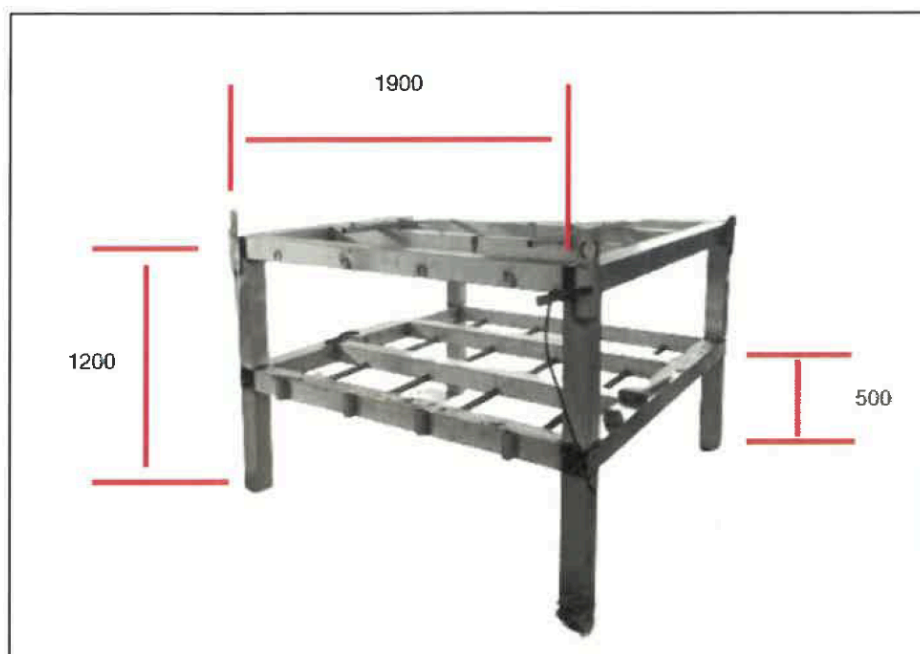
Figura 1 - Struttura portante in acciaio inox e relative dimensioni (misure in mm)
