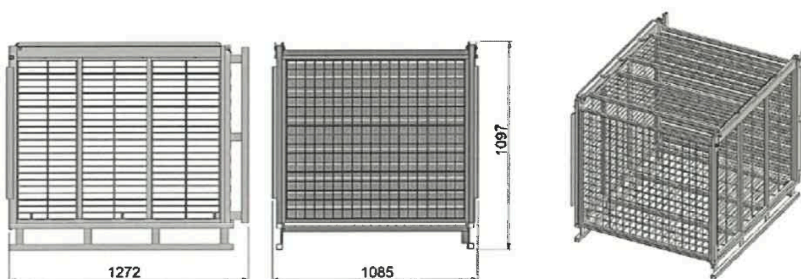
Figura 2 – Gabbie in acciaio zincato per il contenimento delle bottiglie di vino
