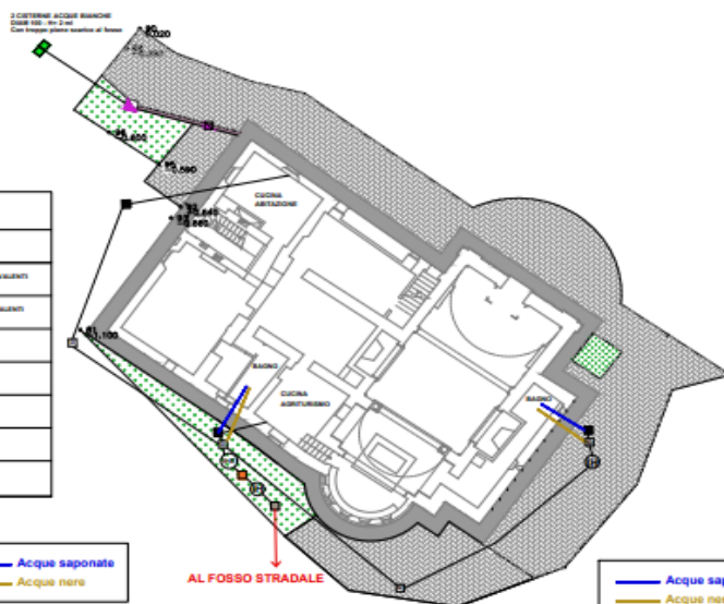
PIANO PRIMO
