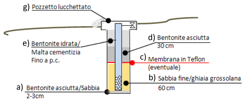
Figura 7: Schema riempimento intercapedine foro-sonda
